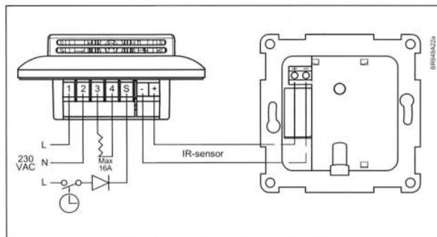
Схема подключения
